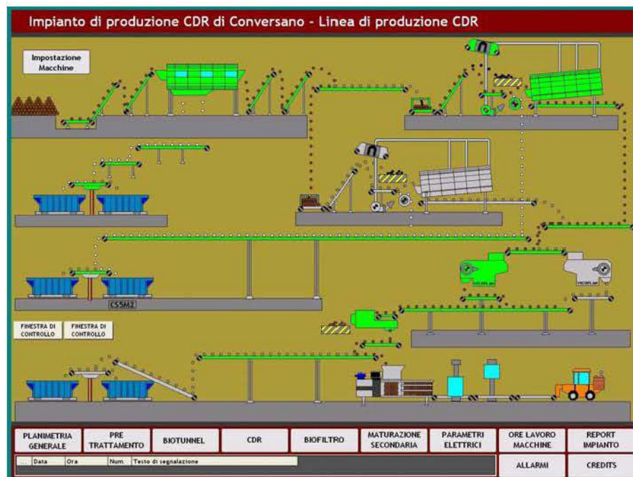
Figura 5 - schermata Lay out Produzione CDR/CSS
