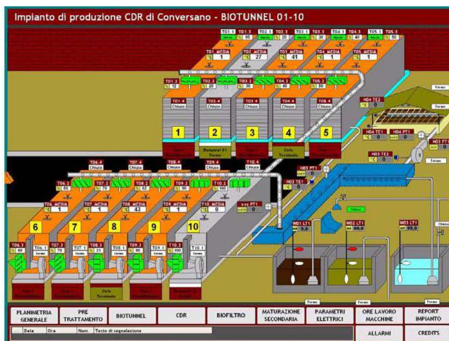
Figura 4 - schermata Lay out
